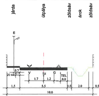
nyílt árokkal
