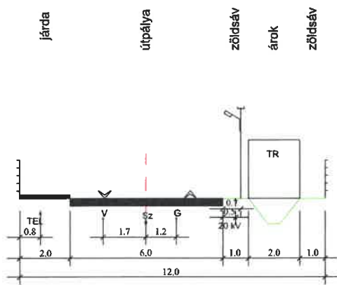
nyílt árokkal
