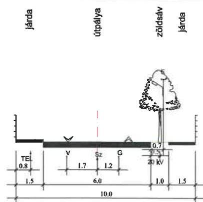
zárt csapadékcsatornával
