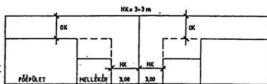
TŰZFAL NÉLKÜLI KIALAKÍTÁS
