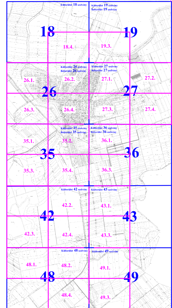
1:2000 méretarányú szabályozási terv szelvényezése
