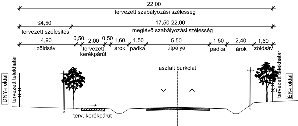
Szélesköz külterületi gyűjtő-összekötőút
