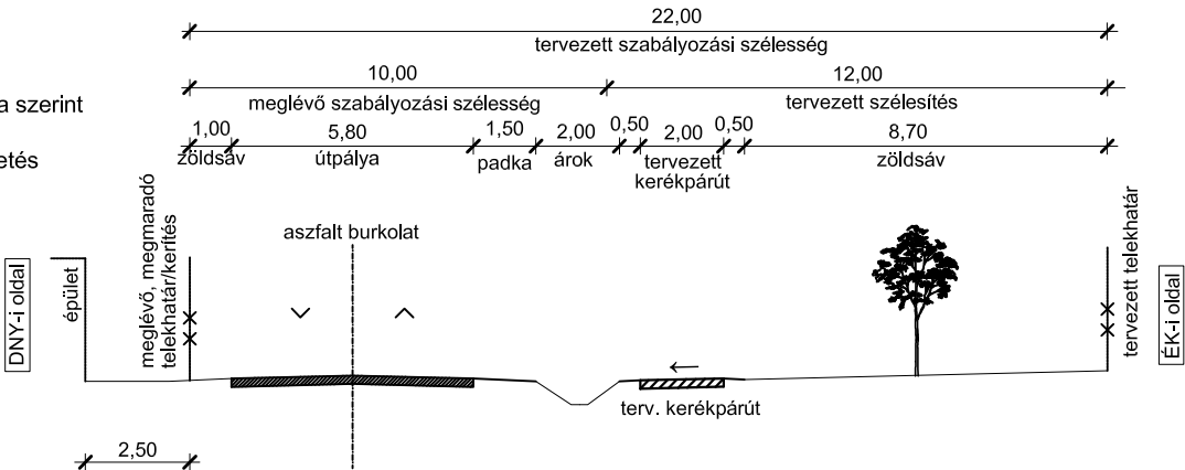
Gazdasági dűlőút külterületi gyűjtő-összekötőút (iparvágány északi vége és a helveciai bekötőút közötti szakasz)
