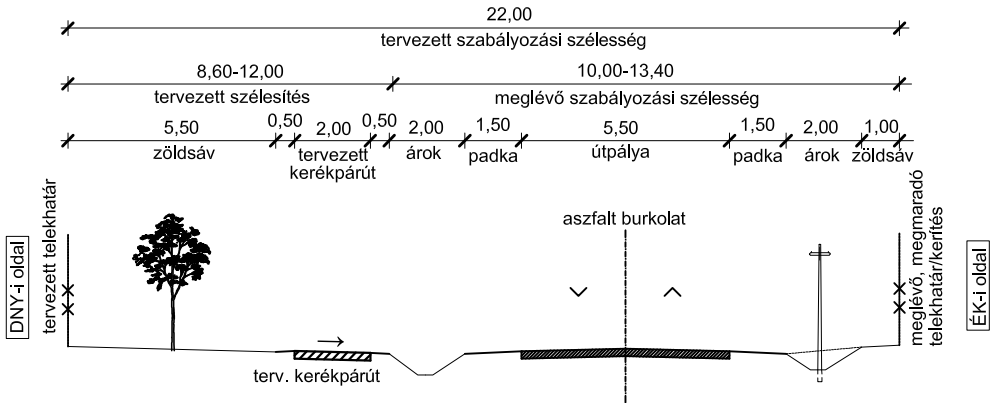
Gazdasági dűlőút külterületi gyűjtő-összekötőút (Kiskőrösi út és az iparvágány északi vége közötti szakasz)
