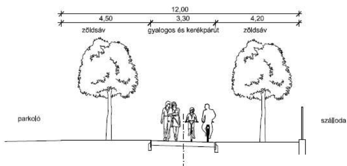
Tervezett gyalogos és kerékpárút mintakeresztmetsze 12 m szabályozási szélességgel
