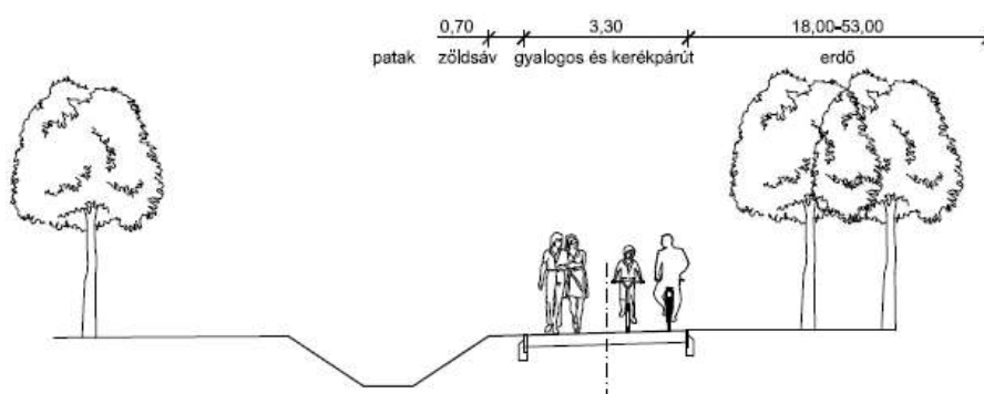
Lenti patak mellett vezetett tervezett gyalogos és kerékpárút mintakeresztmetsze
