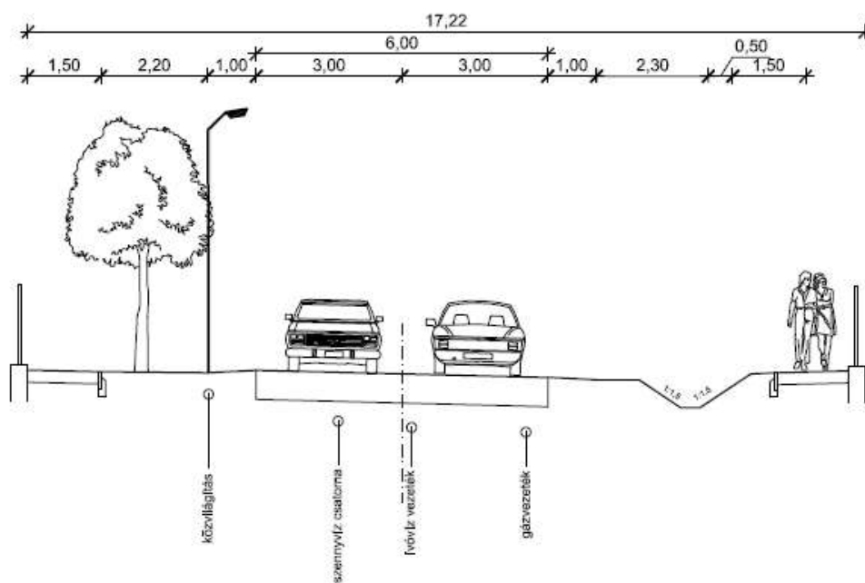
Faluslas lakóterület feltáró útjának mintakeresztmetsze
