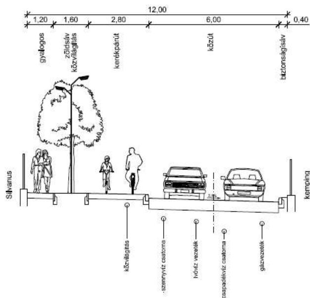
Tervezett 1. sz. út mintakeresztmetsze 12 m szabályozási szélességgel
