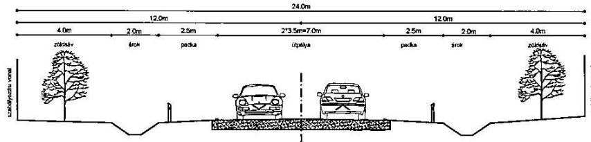
3 jelű mintakeresztmetszvény K.IV. (KÖu-4, KÖu-5) Országos főutak költérületi szakaszai
