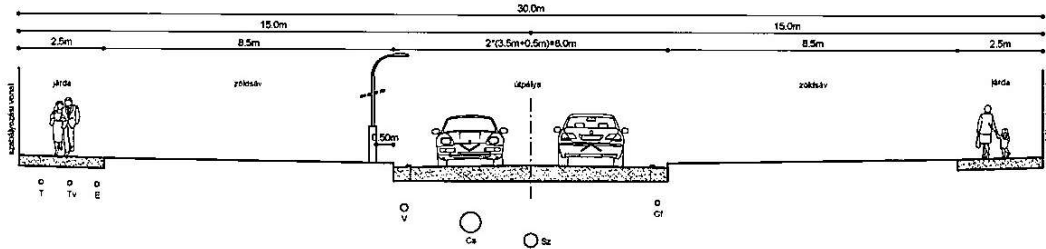
2 jelű mintakeresztmetszvény B.III. (KÖu-3) Országos főutak belterületi szakaszai
