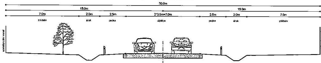
1 jelű mintakeresztmetszvény K.III. (KÖu-3) Országos főutak költérületi szakaszai
