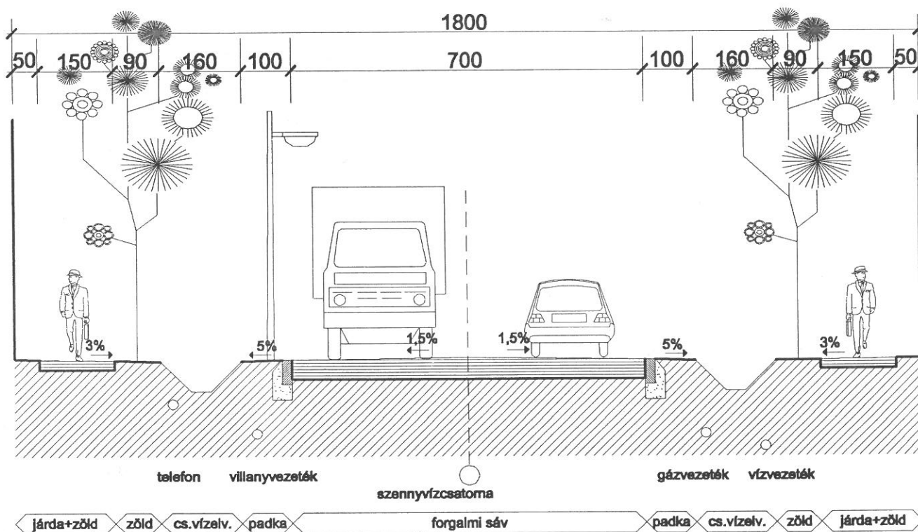
2. mintaszelvény - Márkus-Halastó összekötőút belterületi szakasza szabályozási szélesség: 18,0 m
