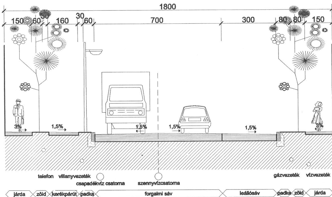
2. mintaszelvény - Márkus-Halastó összekötőút belterületi szakasza szabályozási szélesség: 18,0 m
