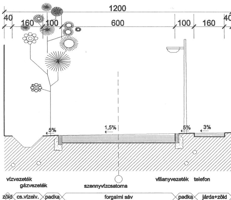
6. mintaszelvény - Üdülőterület útjai szabályozási szélesség: 12,0 m
