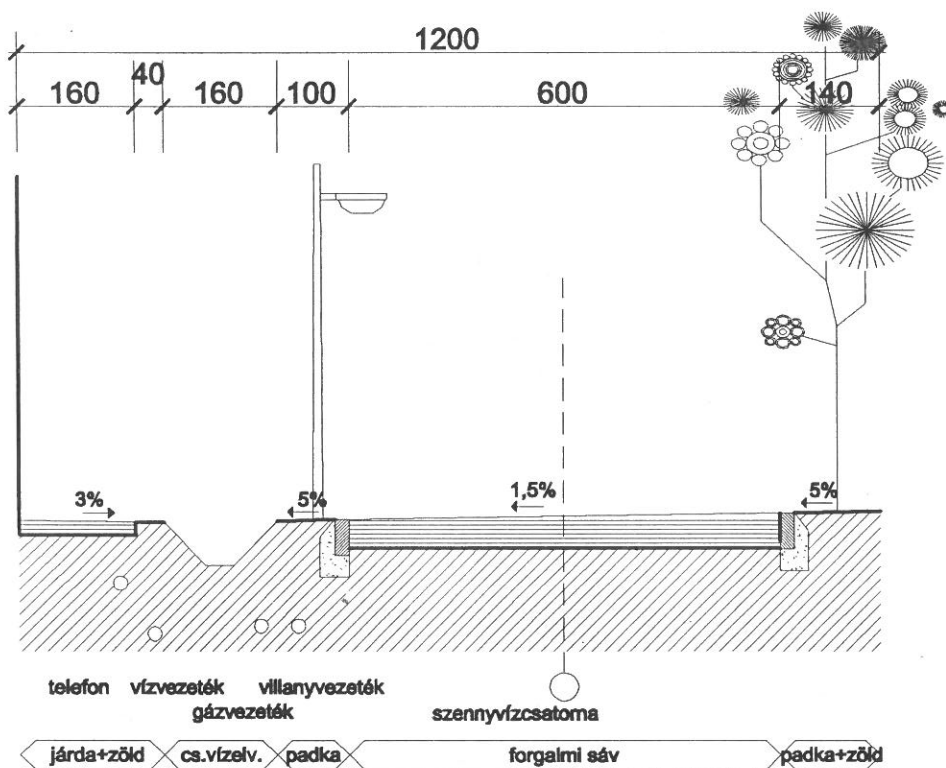
6. mintaszelvény - Üdülőterület útjai szabályozási szélesség: 12,0 m
