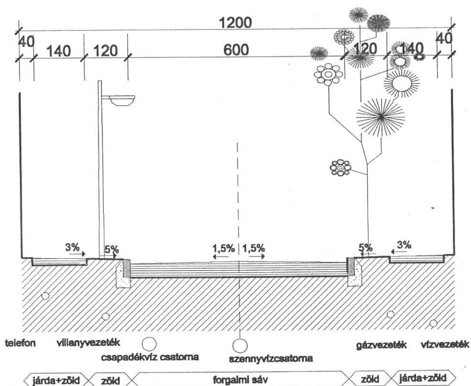
4. mintaszelvény - Ady Endre utca szabályozási szélesség: 12,0 m
