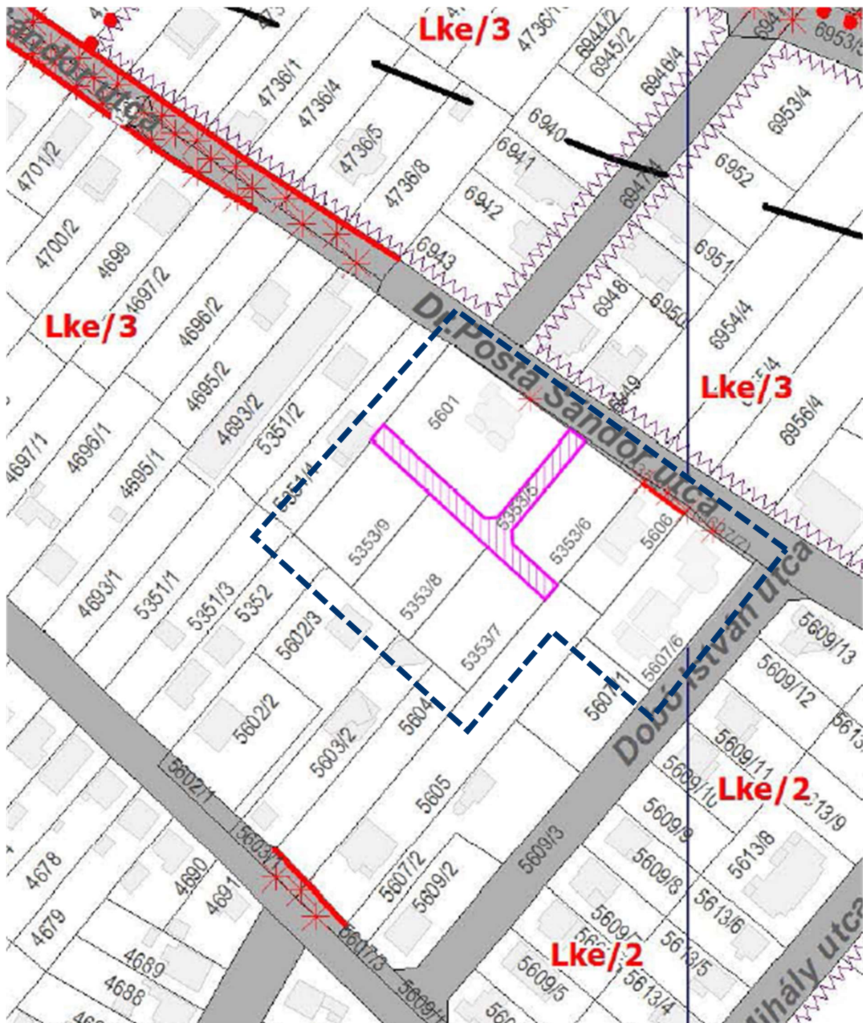
DUNAHARASZTI VÁROS SZABÁLYOZÁSI TERV B-3 ÉS C-3 JELŰ ÉS SORSZÁMÚ TERVLAPJÁNAK MÓDOSÍTÓ RÉSZLETE
