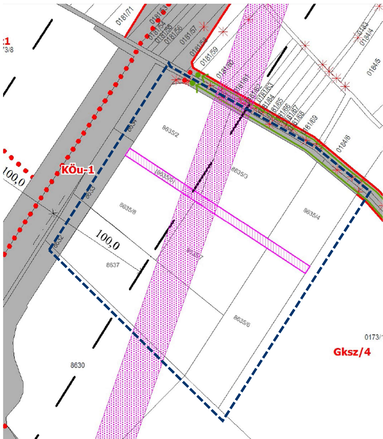
DUNAHARASZTI VÁROS SZABÁLYOZÁSI TERV C-7 JELŰ ÉS SORSZÁMÚ TERVLAPJÁNAK MÓDOSÍTÓ RÉSZLETE
