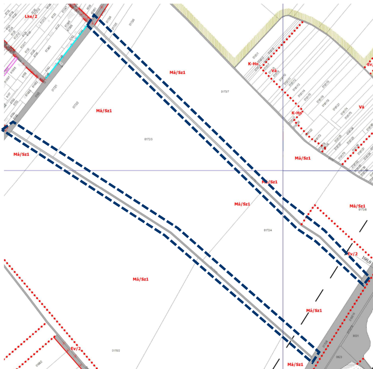
DUNAHARASZTI VÁROS SZABÁLYOZÁSI TERV B-6, B-7 ÉS C-6 JELŰ ÉS SORSZÁMÚ TERVLAPJÁNAK MÓDOSÍTÓ RÉSZLETE
