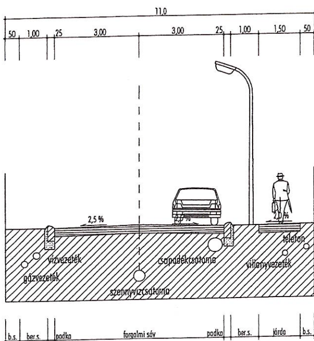
Belterületi utak mintaszelvénye A tervezett Kistrákosra vezető összekötő út és a Keleti utca csomópontja szabályozási szélesség: 11,0 m
