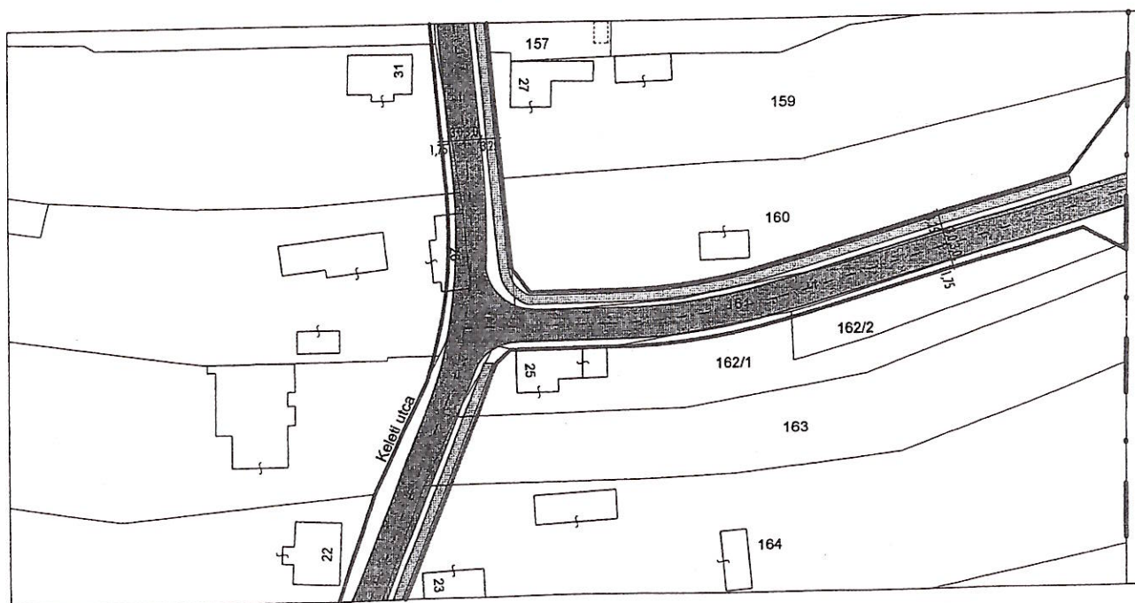
Belterületi utak mintaszelvénye A tervezett Kistrákosra vezető összekötő út és a Keleti utca csomópontja szabályozási szélesség: 11,0 m
