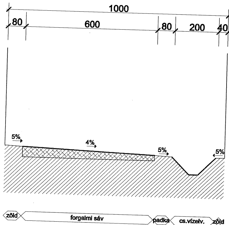
mezőgazdasági út egyoldali vízelvezetéssel szabályozási szélesség: 10,0 m
