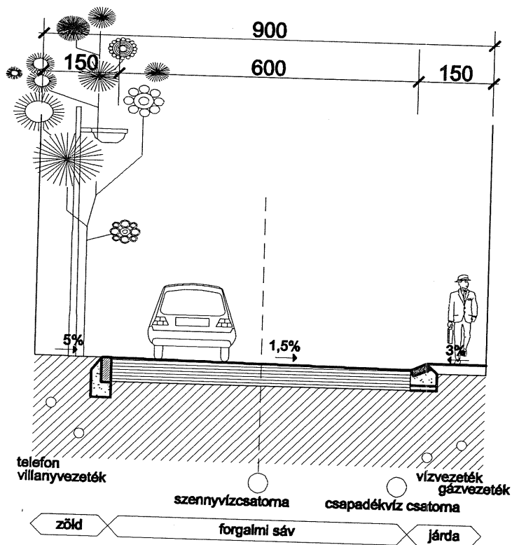
kiszolgáló utak mintaszelvénye szabályozási szélesség: 9,0 m
