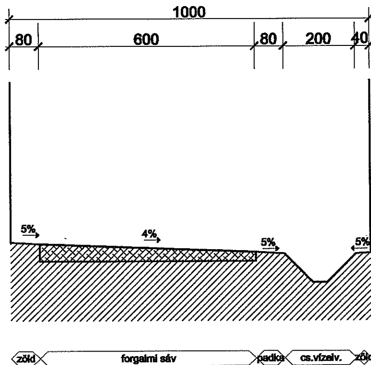
mezőgazdasági út egyoldali vízvezetéssel szabályozási szélesség: 10,0 m
