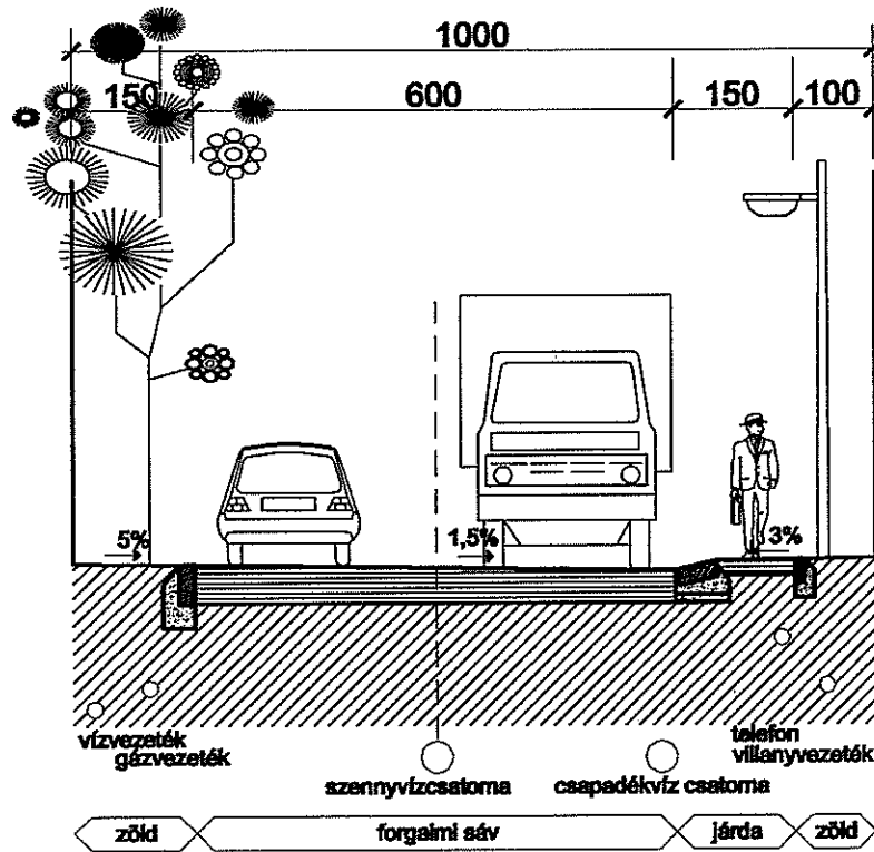
kiszolgáló utak mintaszelvénye szabályozási szélesség: 10,0 m
