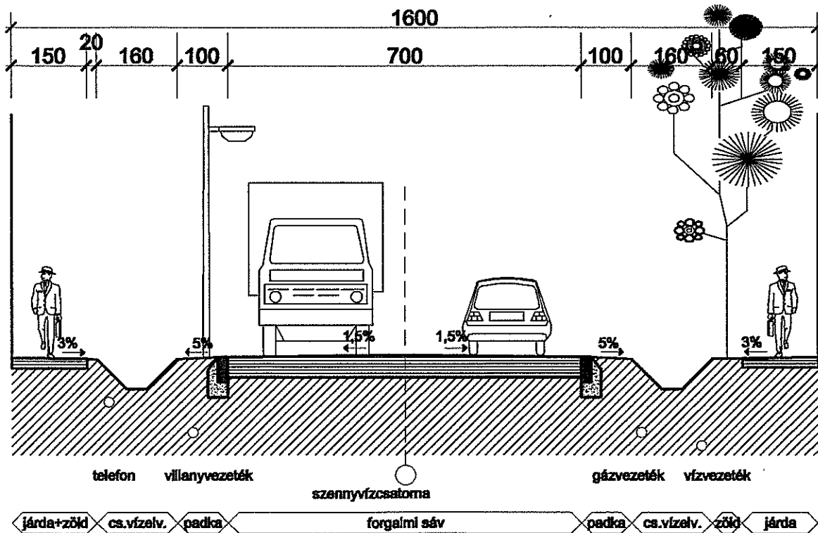
helyi gyűjtőutak mintaszelvénye szabályozási szélesség: 16,0 m
