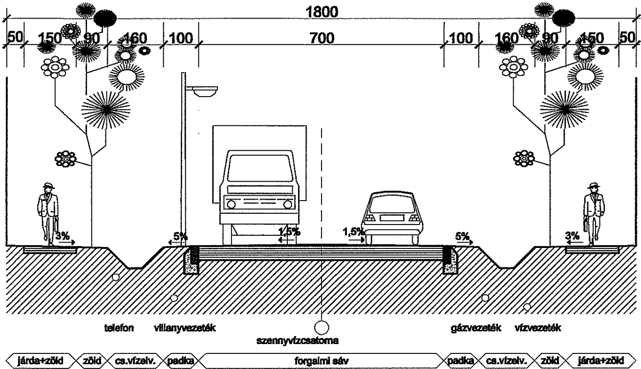
helyi gyűjtőutak mintaszelvénye szabályozási szélesség: 18,0 m
