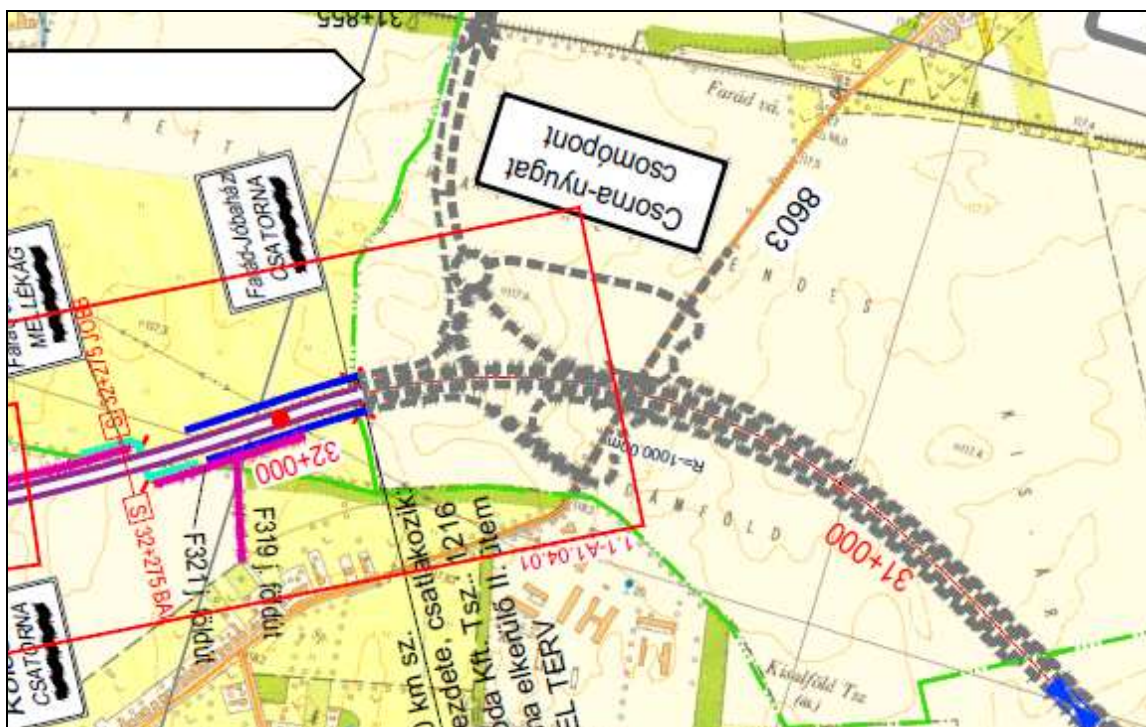
Kivonat a tervezett M85 gyorsforgalmi út nyomvonaltervéből (FÖMTERV Zrt., 2016.11.)
