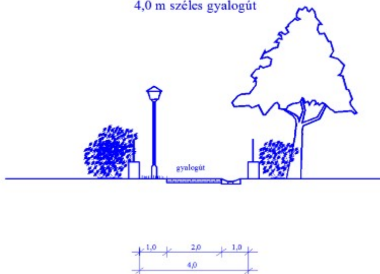
4,0 m széles gyalogút
