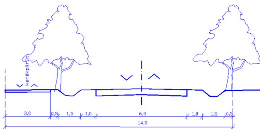
Településközi út kerékpár úttal
