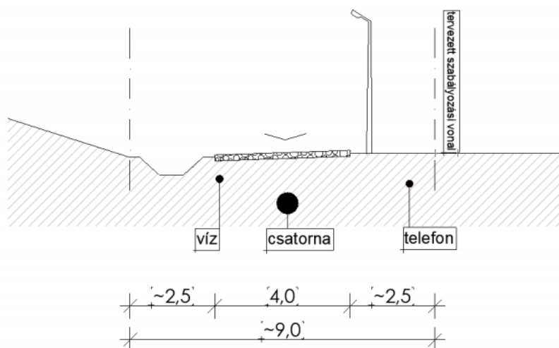
4,7 - 9 méter szabályozási szélességű utak általános mintakeresztmetsze M1:200
