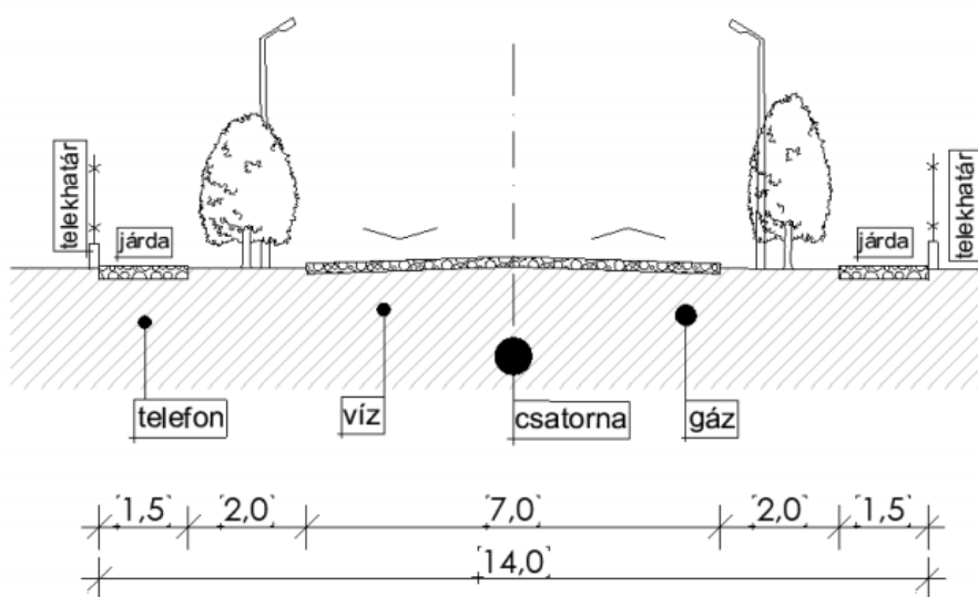
14 méter szabályozási szélességű utak általános mintakeresztmetszvénye M1:100
