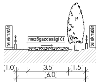
6 méter szabályozási szélességű mezőgazdasági kiszolgálóút mintakeresztmetsze M1:100
