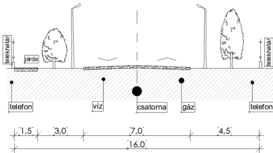
16 méter szabályozási szélességű utak általános mintakeresztmetszvénye M1:100
