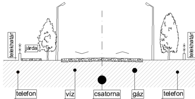
A 12 méter szabályozási szélességű utak általános mintakeresztmetsze M1:100
