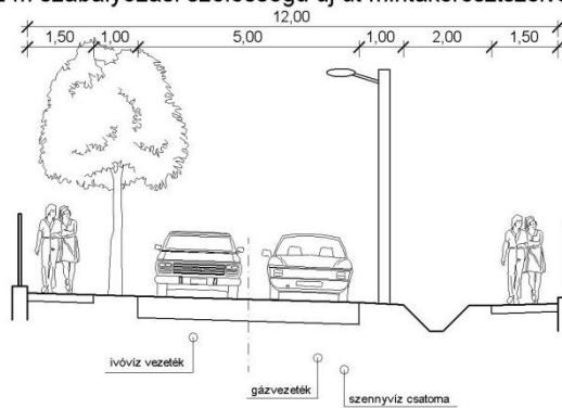
Tervezett 12 m szabályozási szélességű új út mintakeresztmetszelve
