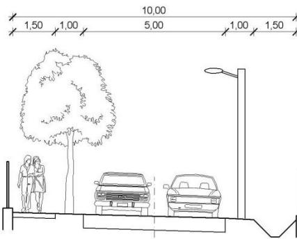
Tervezett 10 m szabályozási szélességű új út mintakeresztmetszelve
