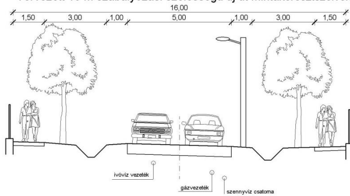
Tervezett 16 m szabályozási szélességű új út mintakeresztmetszelve
