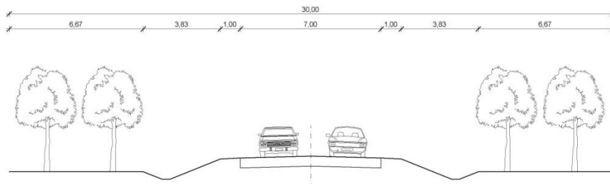
Tervezett elkerülő út mintakeresztmetszelve
