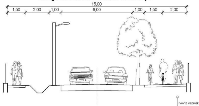
Margaréta utca mintakeresztmetszelve
