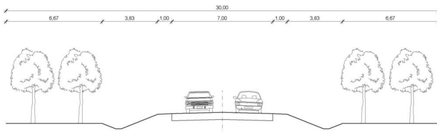
Tervezett elkerülő út mintakeresztmetsze
