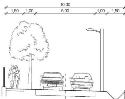
Tervezett 10 m szabályozási szélességű új út mintakeresztelvénye
