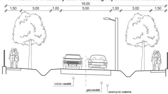
Tervezett 16 m szabályozási szélességű új út mintakeresztmetsze
