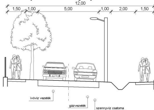
Tervezett 12 m szabályozási szélességű új út mintakeresztelvénye
