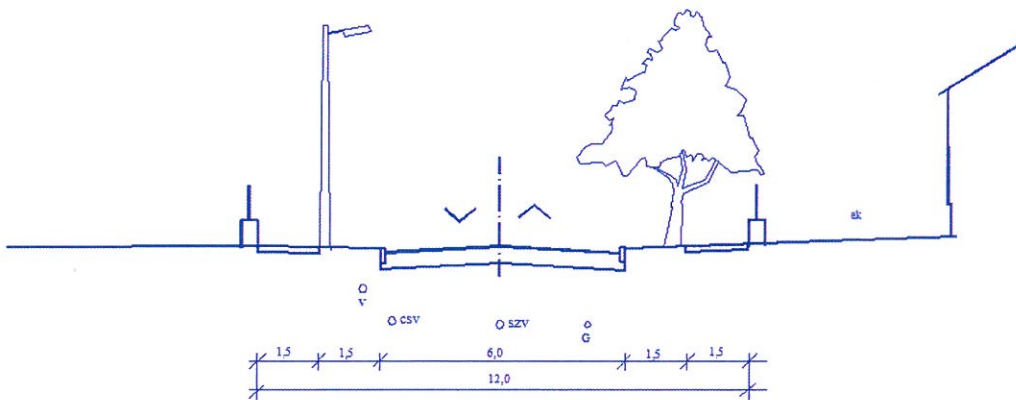
2. Tervezett kiszolgáló út egyoldali beépítéssel
