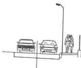
Mucsi 5. Mucsi-Papdi kápolna közti elválasztás nélküli közös gyalog- és kerékpárút mintakeresztmetszele
