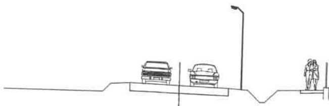
2. Dózsa Gy. út mintakeresztmetszele
