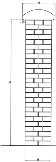
URADALMI KERÍTÉS RAJZA M=1:20 OLDALNÉZET
