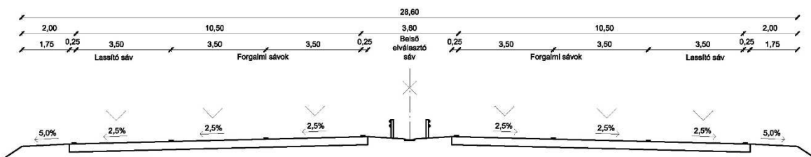
Mintakeresztmetszvény, M25 autót lassító sávokkal
