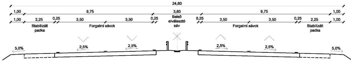
Mintakeresztmetszvény, M25 autót
