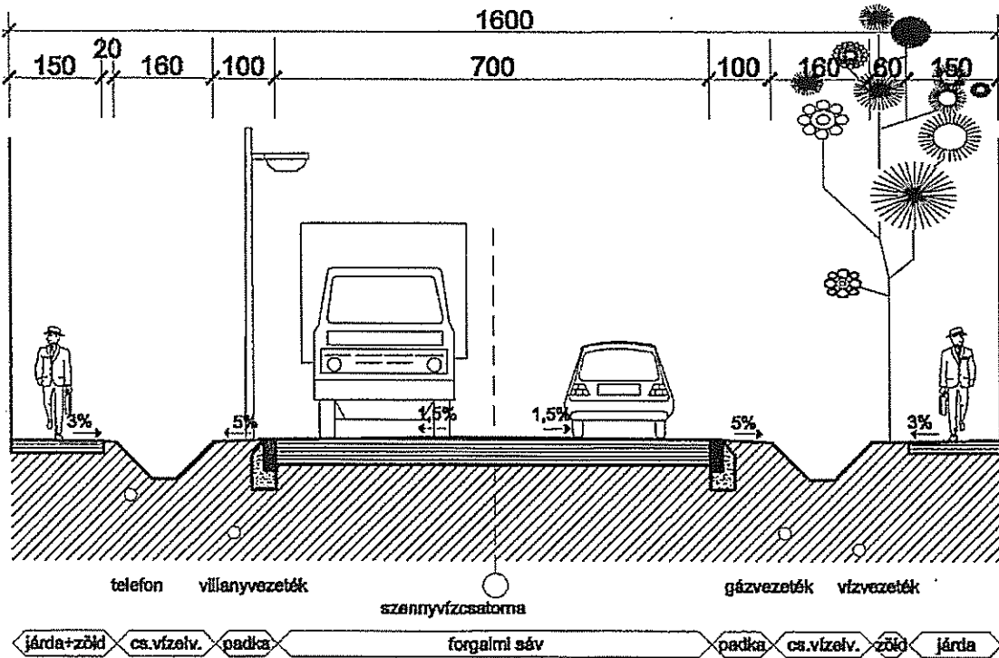
helyi gyűjtőutak mintaszelvénye szabályozási szélesség: 16,0 m
