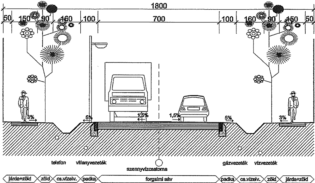
helyi gyűjtőutak mintaszelvénye szabályozási szélesség: 18,0 m
