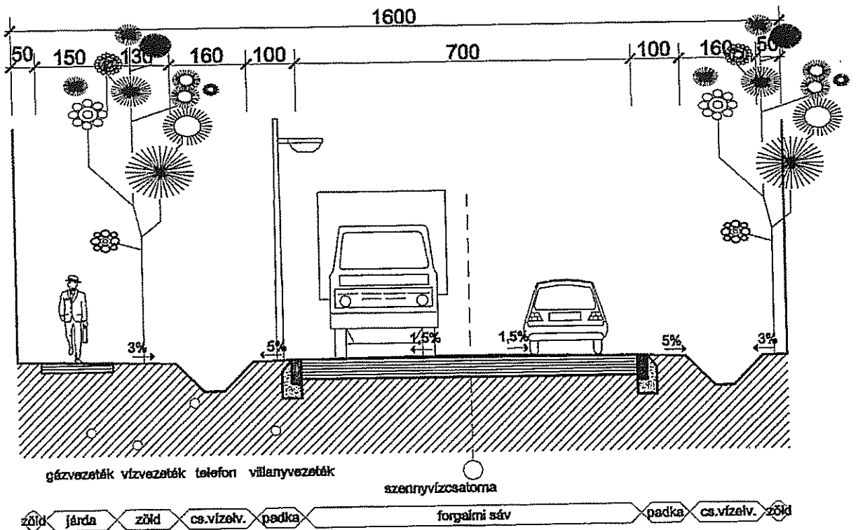
87133. sz. közút Sé belterületi szakaszának mintaszelvénye szabályozási szélesség: 16,0 m
