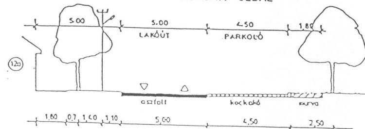
B - B MÁTYÁS TÉR NYUGATI OLDAL
