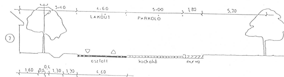
C - C MÁTYÁS TÉR ÉSZAKI OLDAL
