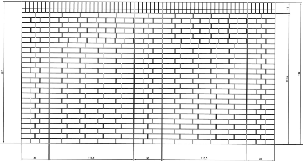
ELŐLNÉZET
