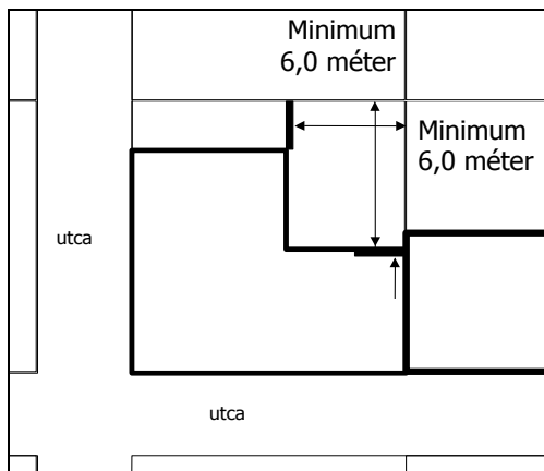
2. ábra: Az épület kialakítása saroktelken, zártsorú beépítési mód esetén
