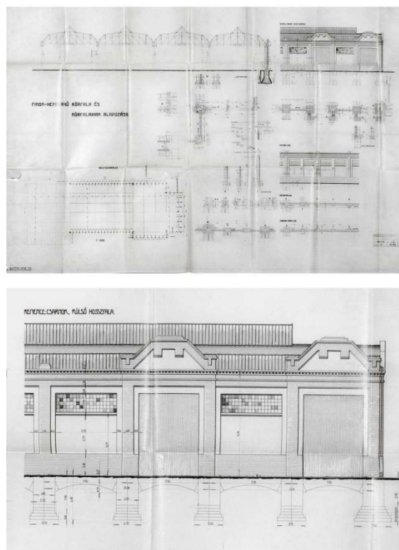
Ózdi Finomhengermű - Tervrajzok - 1912.
