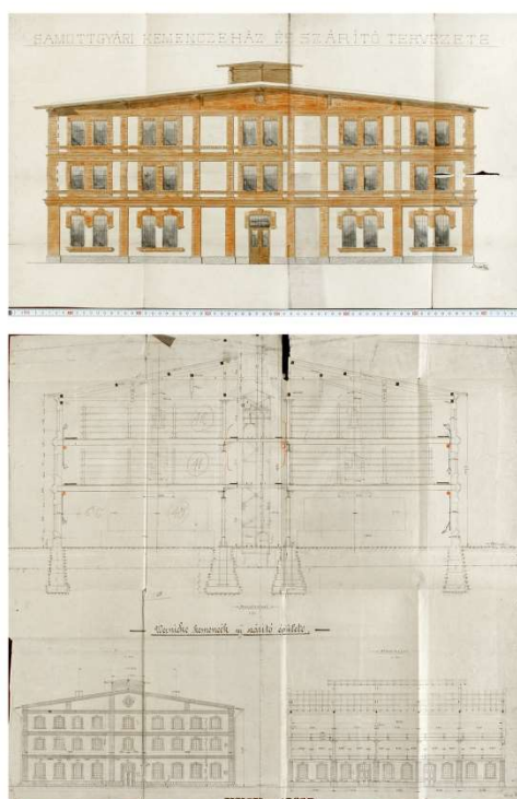
Ózdi Téglagyár - Tervrajzok - 1905.
