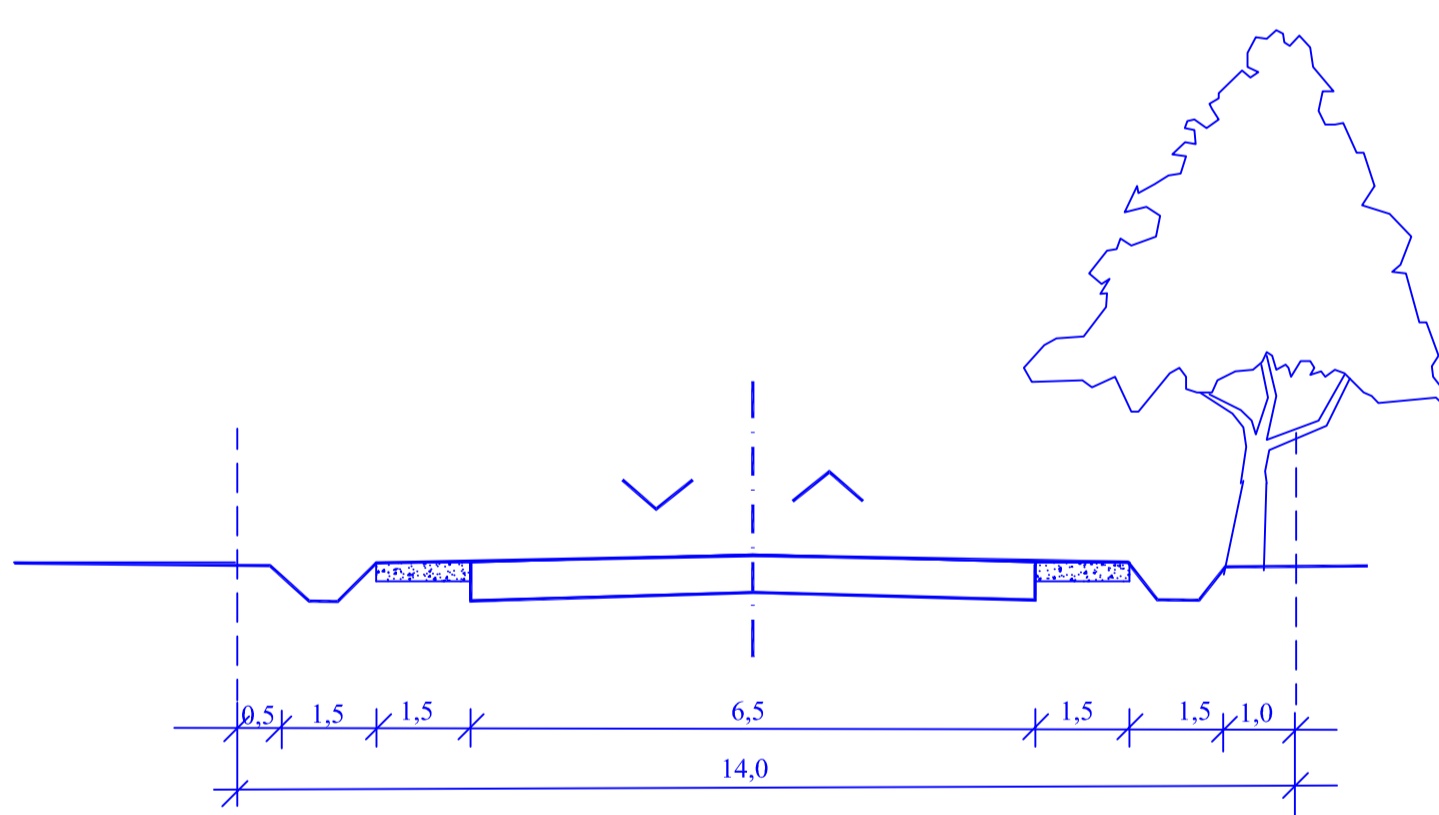
Tervezett országos mellékút K.V.A.90
