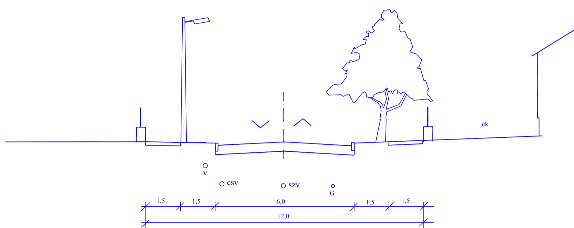
Tervezett kiszolgáló út egyoldali beépítéssel
