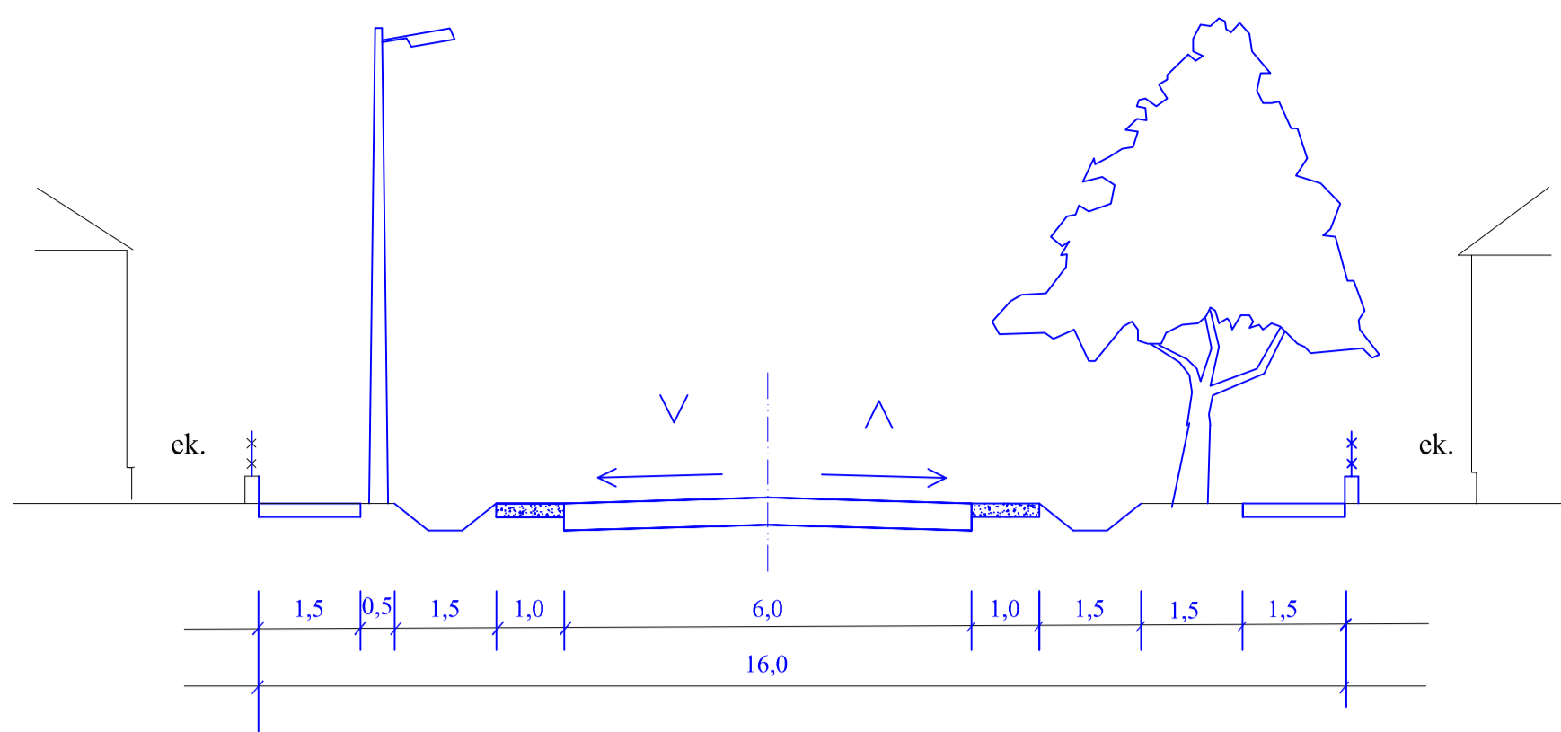
Tervezett kiszolgáló út kétoldali beépítéssel
