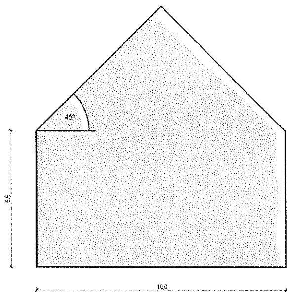
Keresztmetszeti korlát hajlított és utcával párhuzamos gerincű házak utcai szárnyánál
